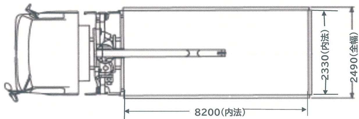
10tユニック車
